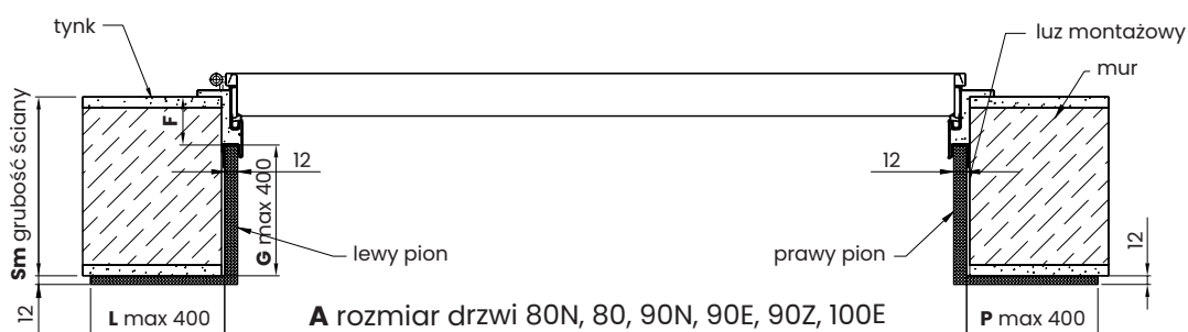
PRZEKRÓJ POZIOMY
